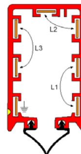
2 paralelno vezana vodiča po fazi
